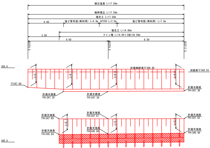
展開図 S=1:100
