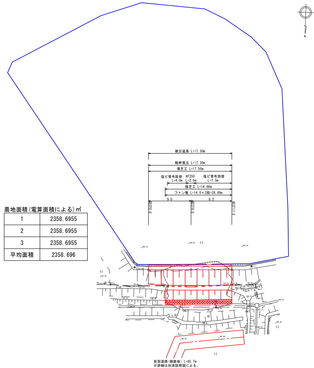
計画平面図 S=1:250
