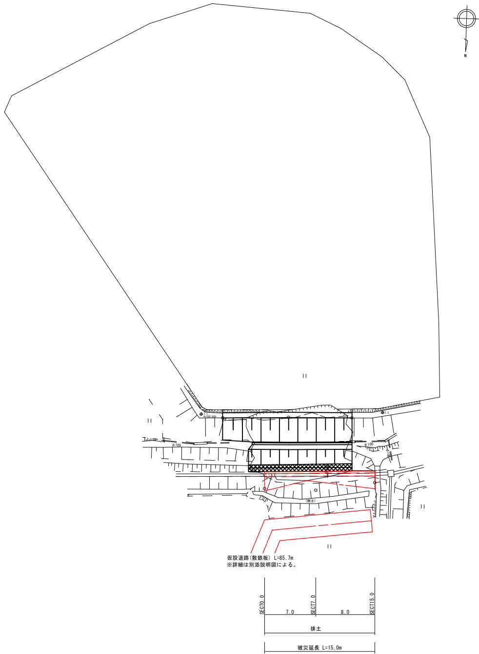
計画平面図 S=1:250
