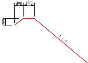
暗渠排水 S=1:20
