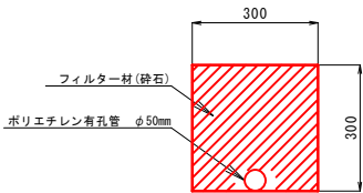
暗渠排水 S=1:20
