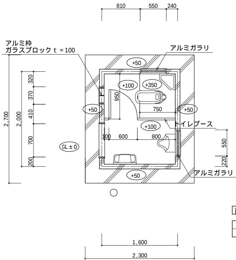
平面図 S=1/50
