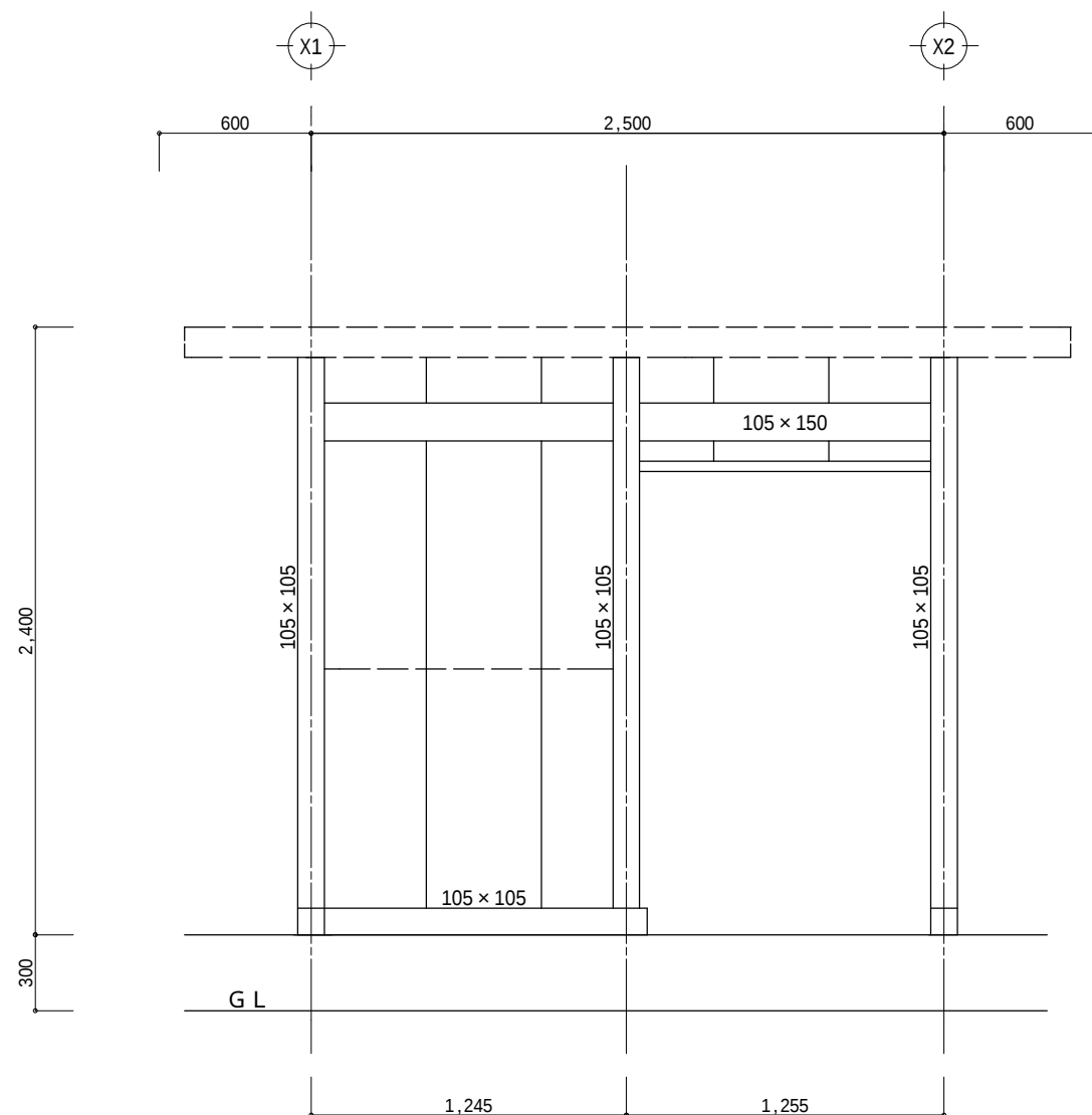
Y1通り軸組図
