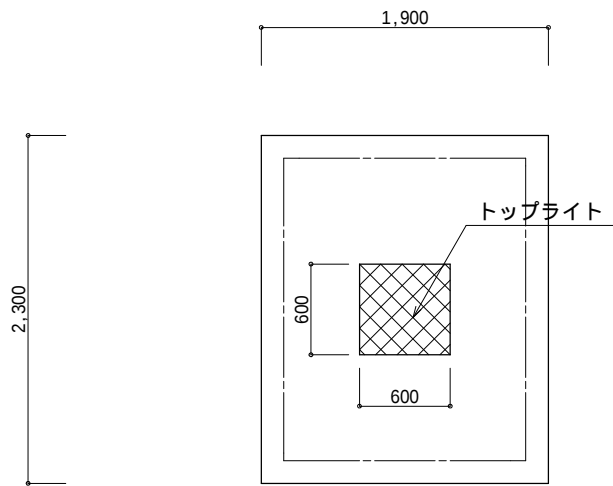
屋根伏図 S=1/50
