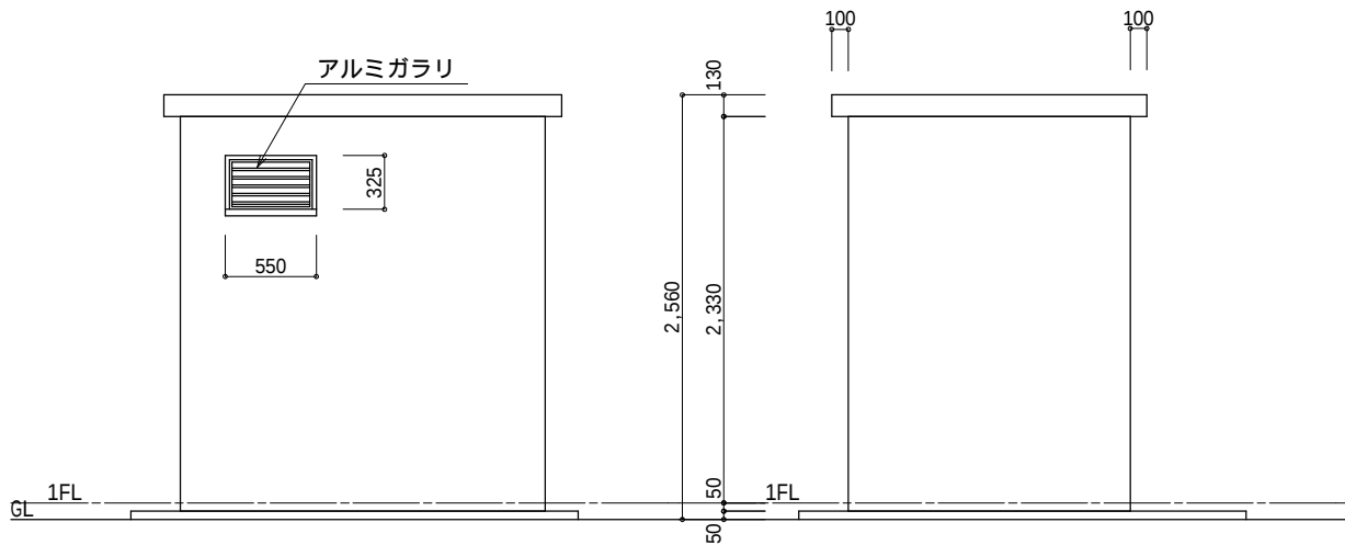
西側立面図 S=1/50
