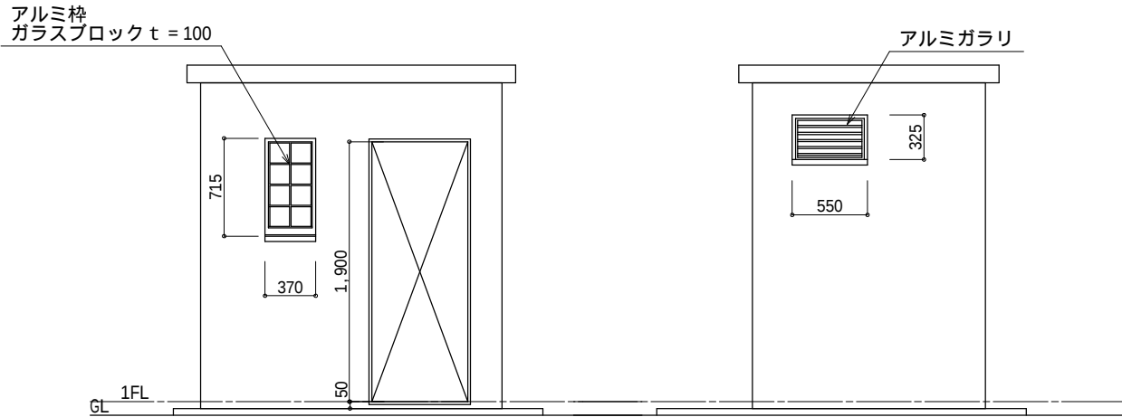
西側立面図 S=1/50
