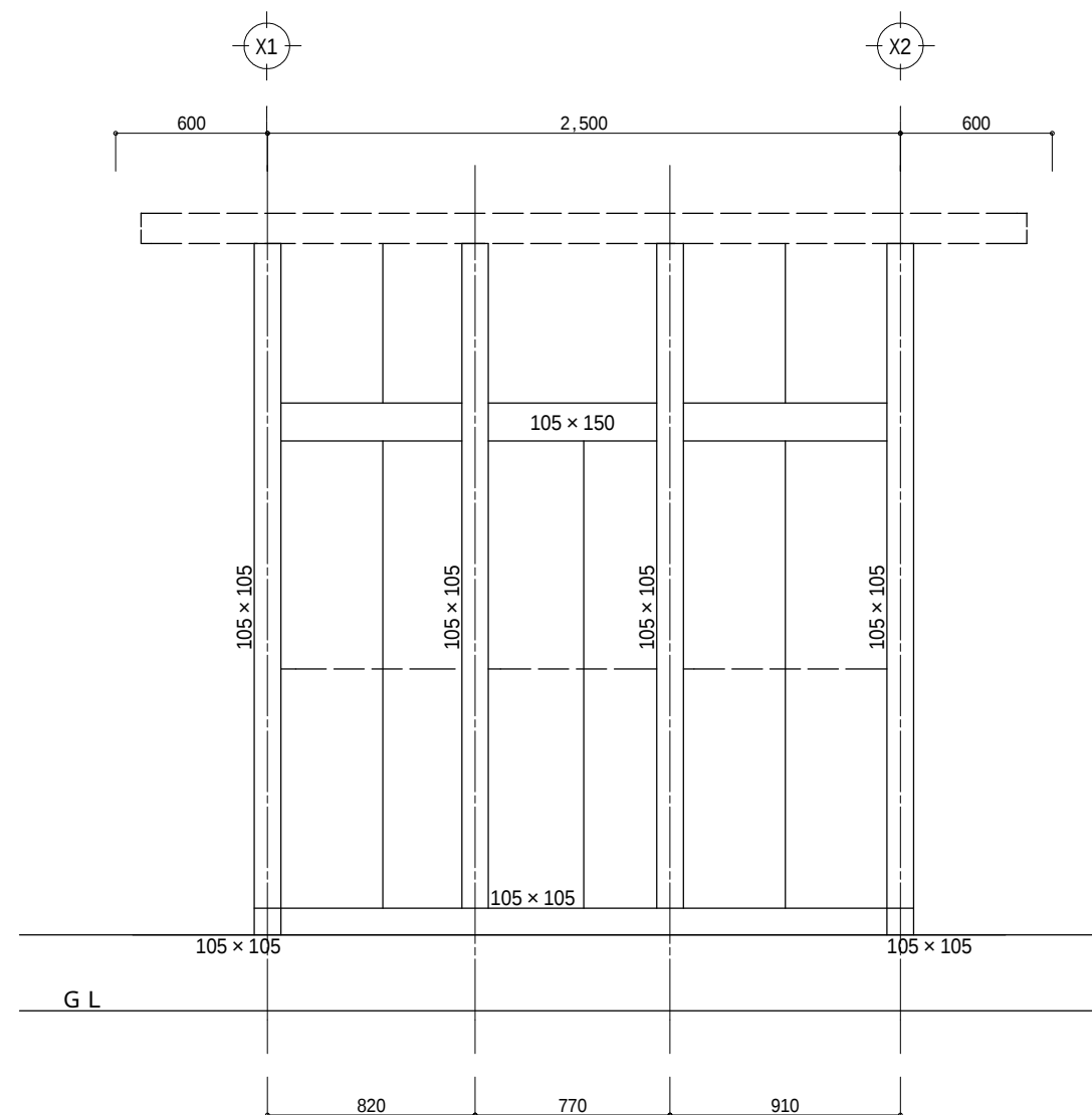
Y2通り軸組図
