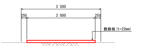
工事用道路 S=1:50
