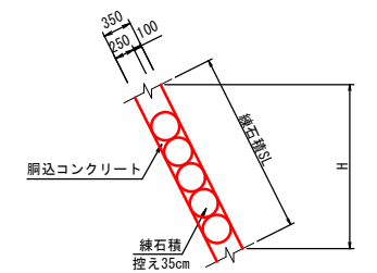
取り付け工 S=1:50
