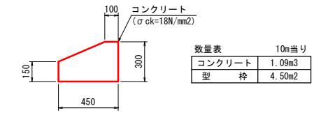
ブロック基礎 S=1:20
