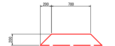
畦畔工 S=1:20
