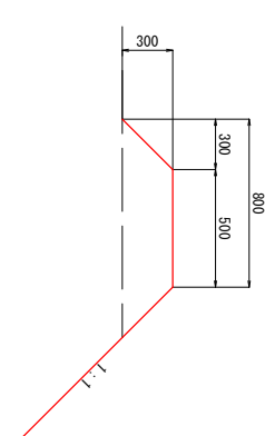
畦畔築立 S=1:25
