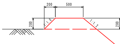
畦畔築立 縮尺=1:20
