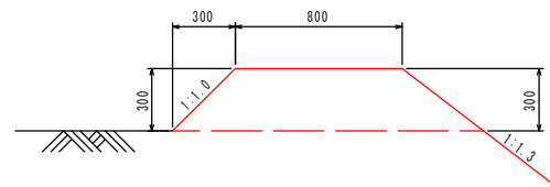
畦畔築立 縮尺=1:20
