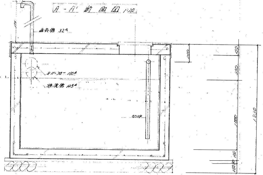
B-B' 断面図 1:20
