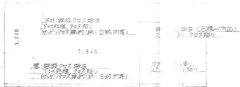
齋場B面展開図 S=1:50
