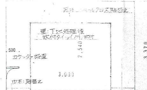
収容室C面展開図 S=1:50
