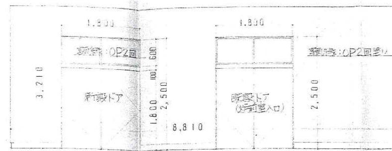
齋場C面展開図 S=1:50
