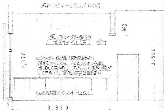
齋場B面展開図 S=1:50
