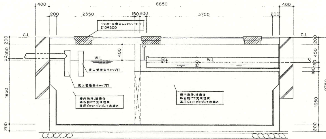
C ~ C' 断面図 縮尺 1:30
