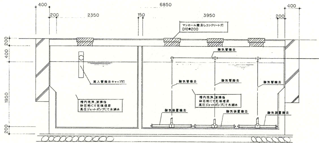
B ~ B' 断面図 縮尺 1:30
