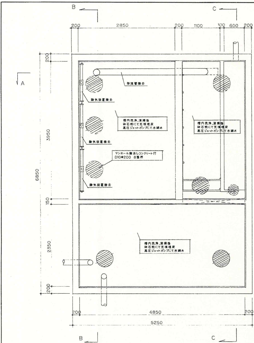
平面図 縮尺 1:30
