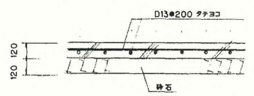
土間復旧図
