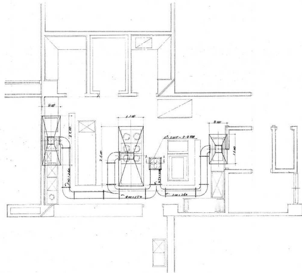
厨房设备安装图
