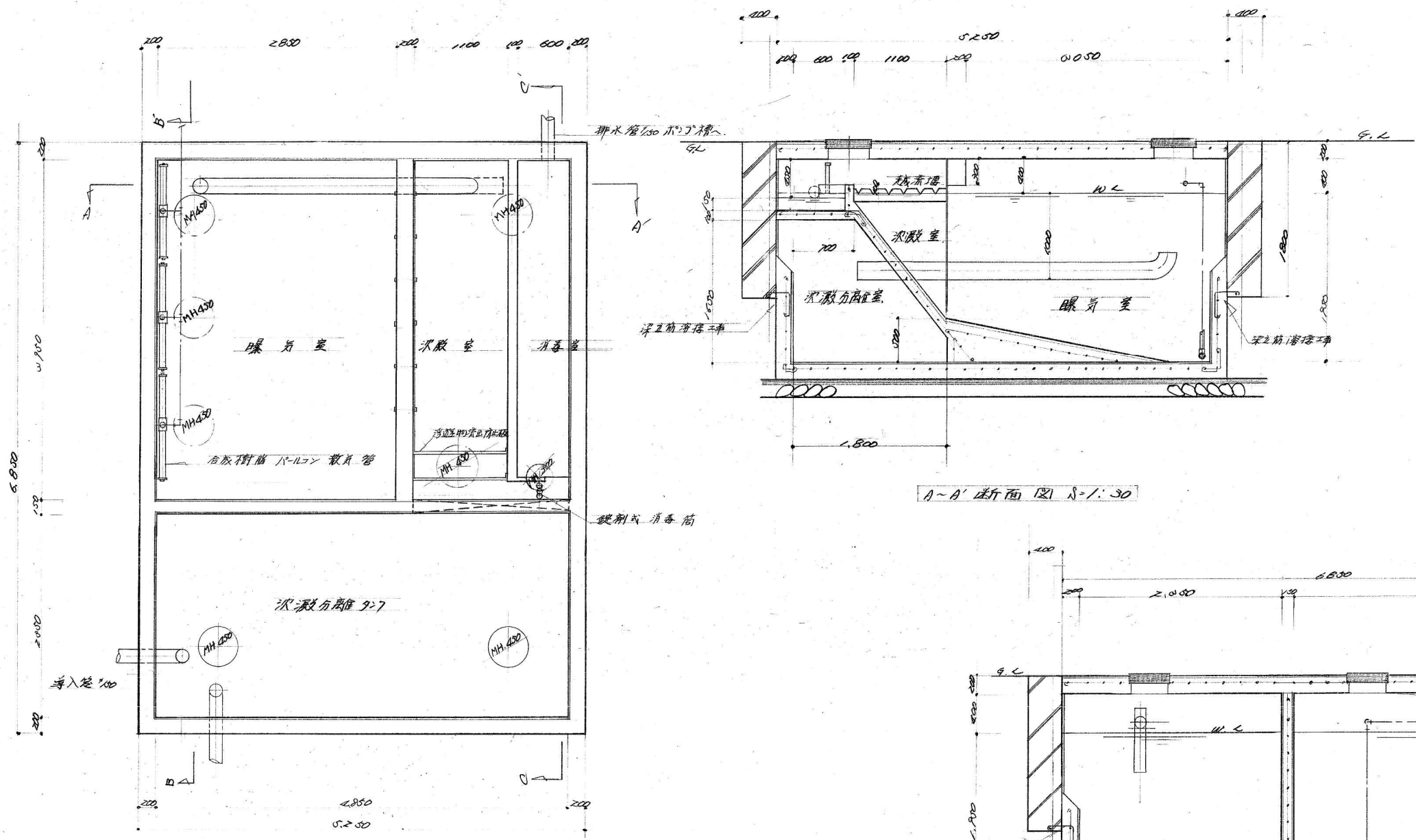
平面图 1:30
