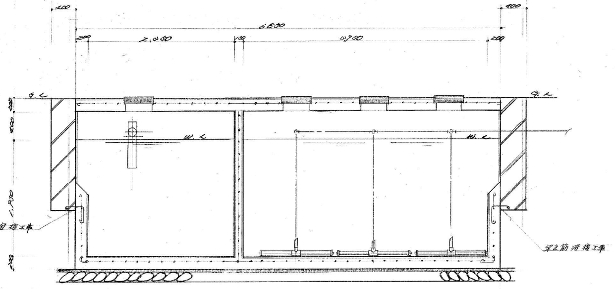
A-A' 断面图 1:30
