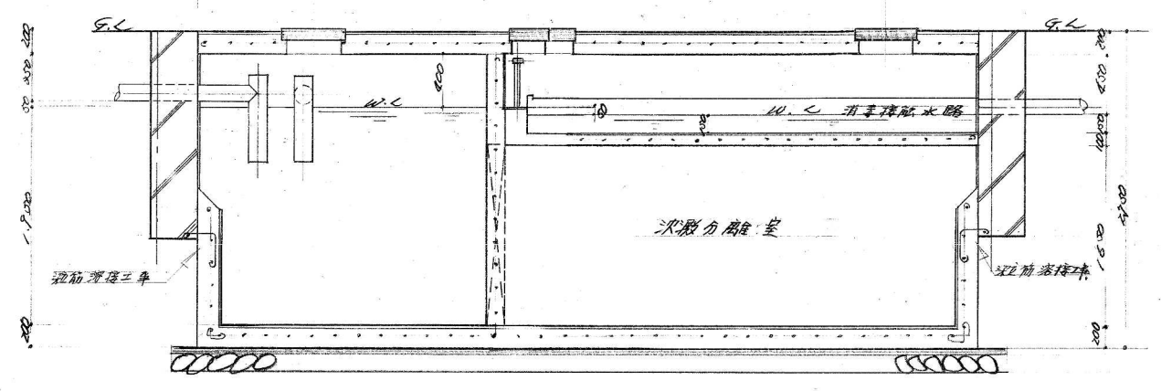
C-C' 断面图 1:30
