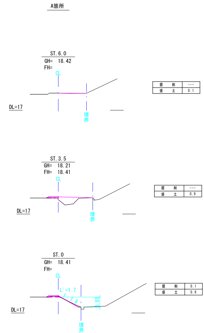
横断図 S=1:100
